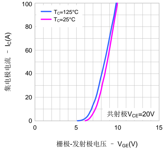
图2. 传输特性
