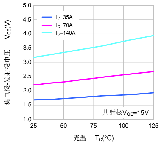
图6. 饱和电压 vs. 壳温
